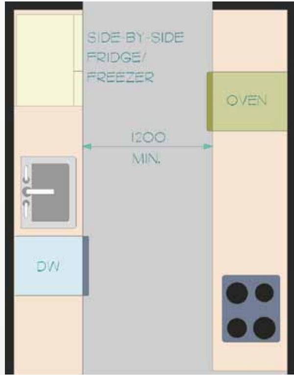
شكل ١٦٢: مطبخ ممكن المرور منه
