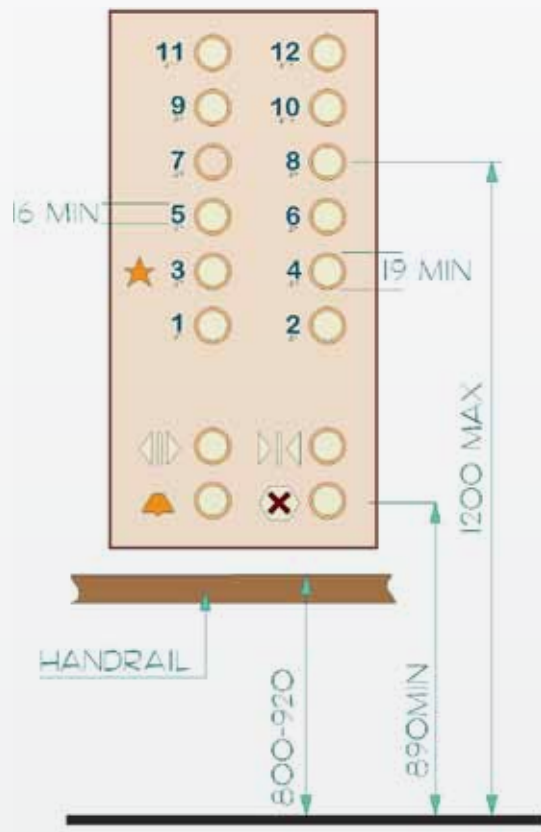
شكل ١٠٦: لوحة التحكم
