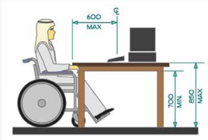
شكل ٢٢٧: أسطح العمل
