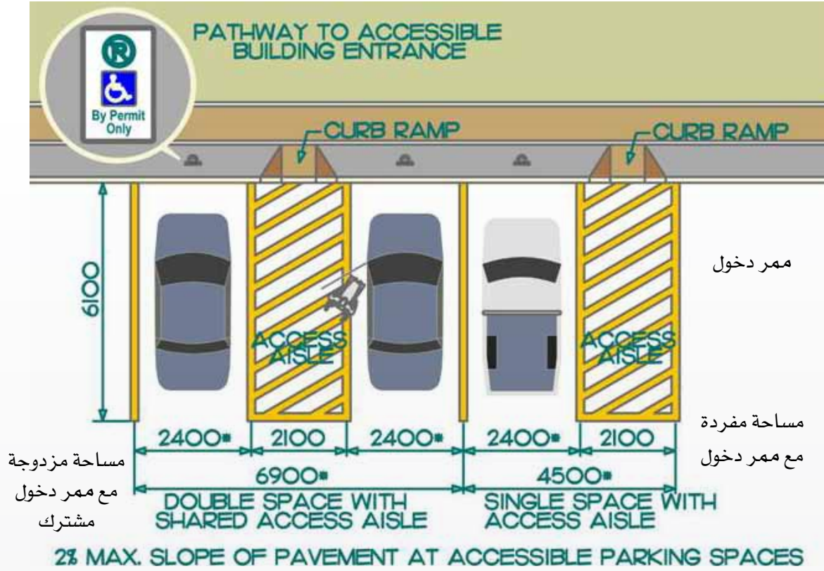
شكل ٧٢: المواقع العمودية
