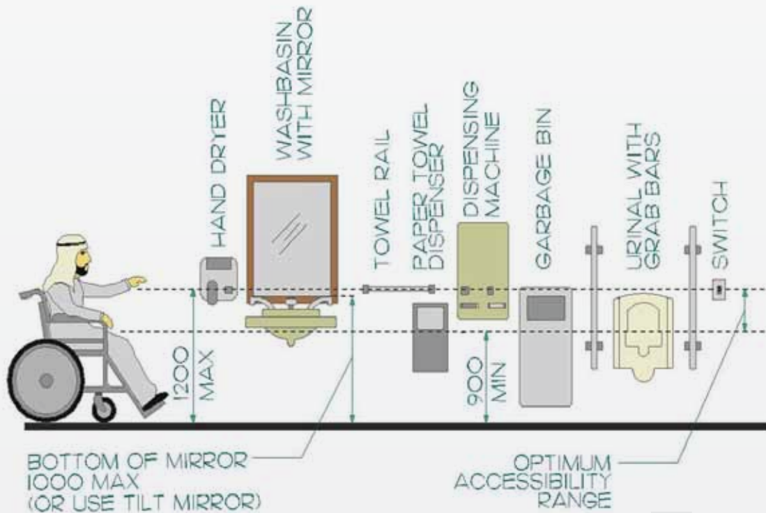
شكل ١٥٣: كماليات الحمام
