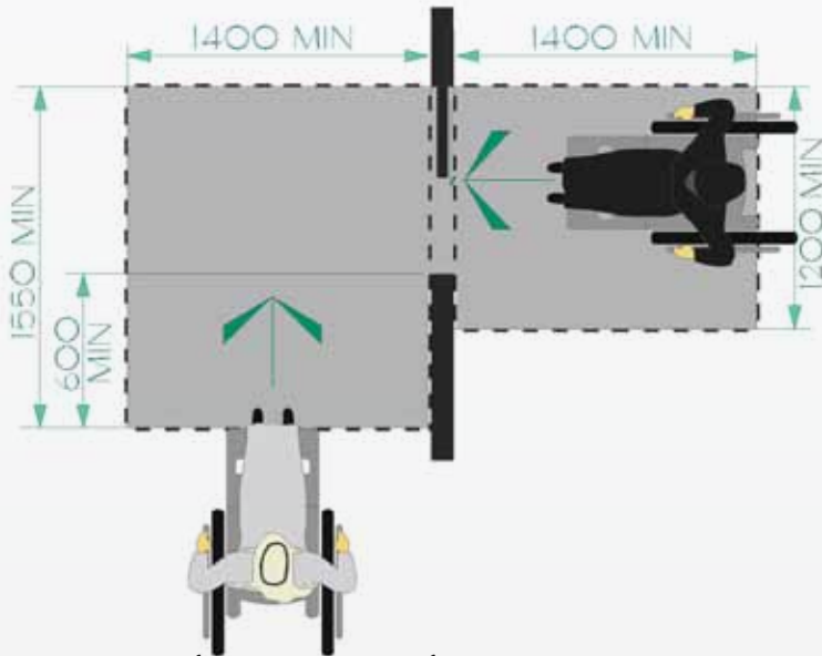
شكل ١١٩: الإقتراب من الأمام والجانب عند الأبواب المنزقة
