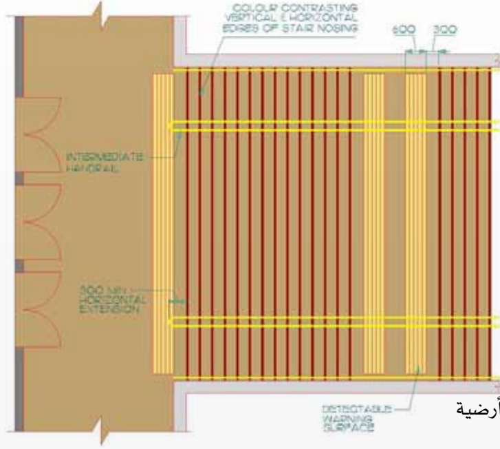
شكل رقم ٥٣: معايير تصميم الدرج
