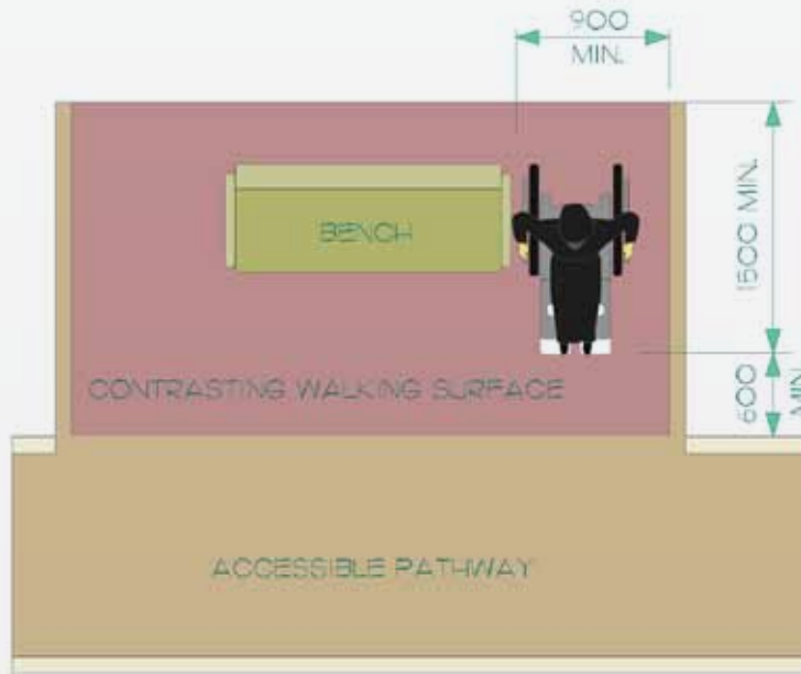
شكل ١٩٤: منطقة الاستراحة
