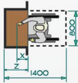
شكل رقم ٢١: فراغ الوصول الأمامي فوق عائق
