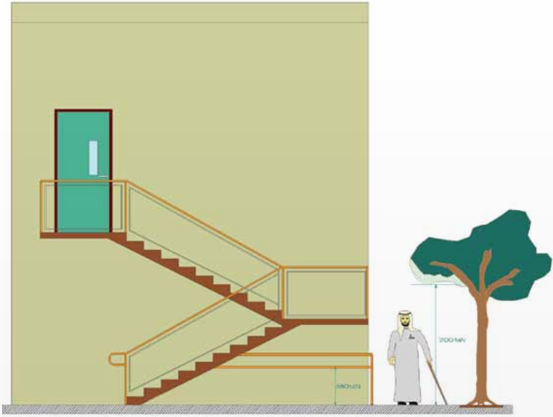
شكل ١٧٩: العوائق
