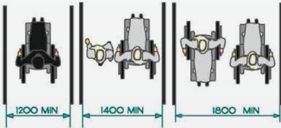
شكل رقم ٤٦: اتساع (عرض) الوصول
