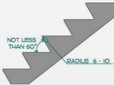
شكل رقم ١٠١: شفة الدرج
