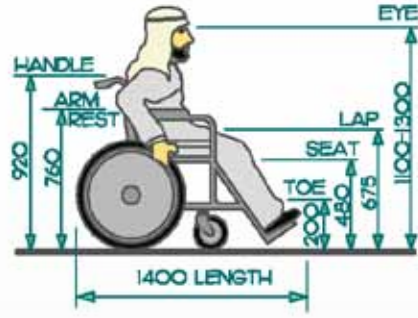
شكل رقم ٢٣: الفراغات الخاصة بكرسي متحرك يدوي خاص بالبالغين
