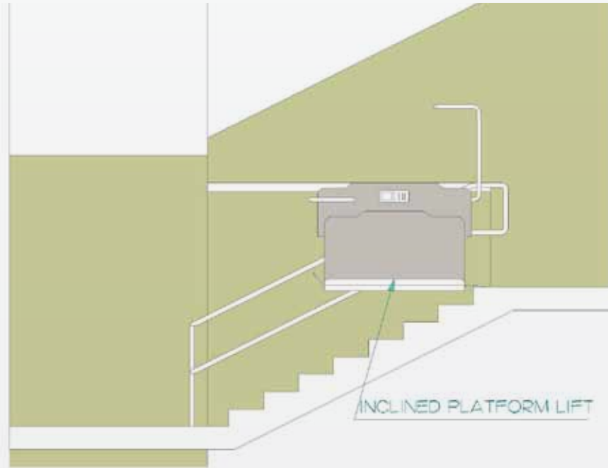
شكل ١١٠: مصعد LA المنحدرة / مصعد السلالم المنحدرة
