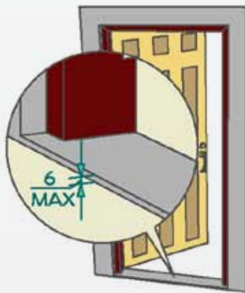
شكل ١٢٢: عتبة الباب
