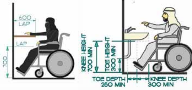
شكل رقم ٢٥: الفراغات الخاصة بالجزء السفلي
