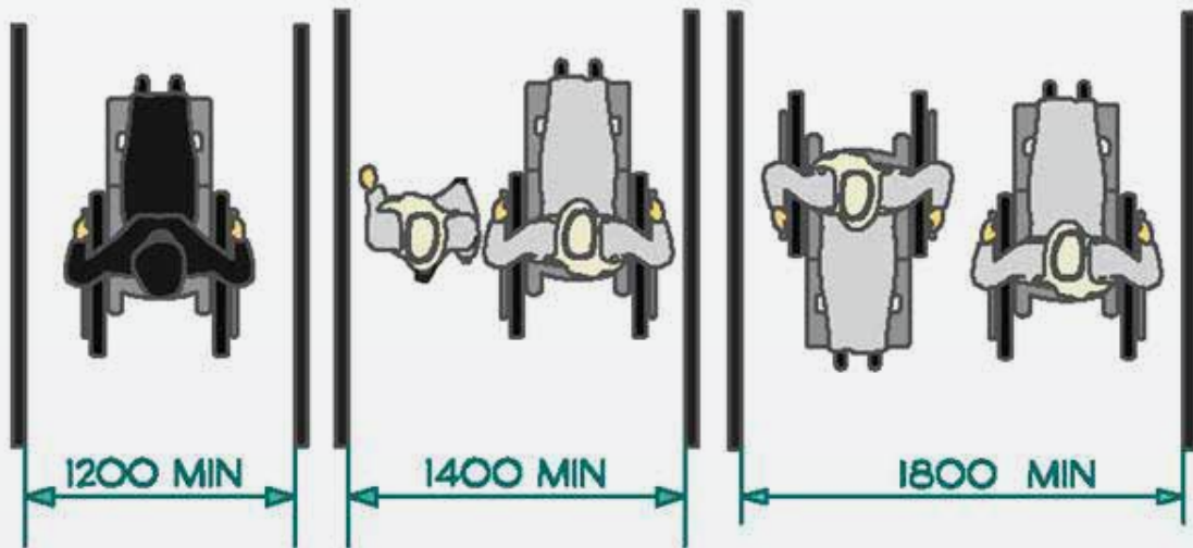
شكل ٩٢: قياسات مختلفة لعرض الوصول
