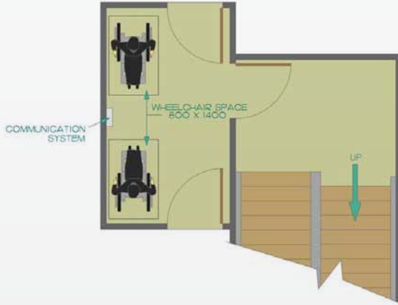
شكل ٢٢١: الرواق المحمي
