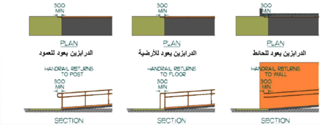
شكل رقم ٤٩: الإمتدادات الأفقية للدرازين
