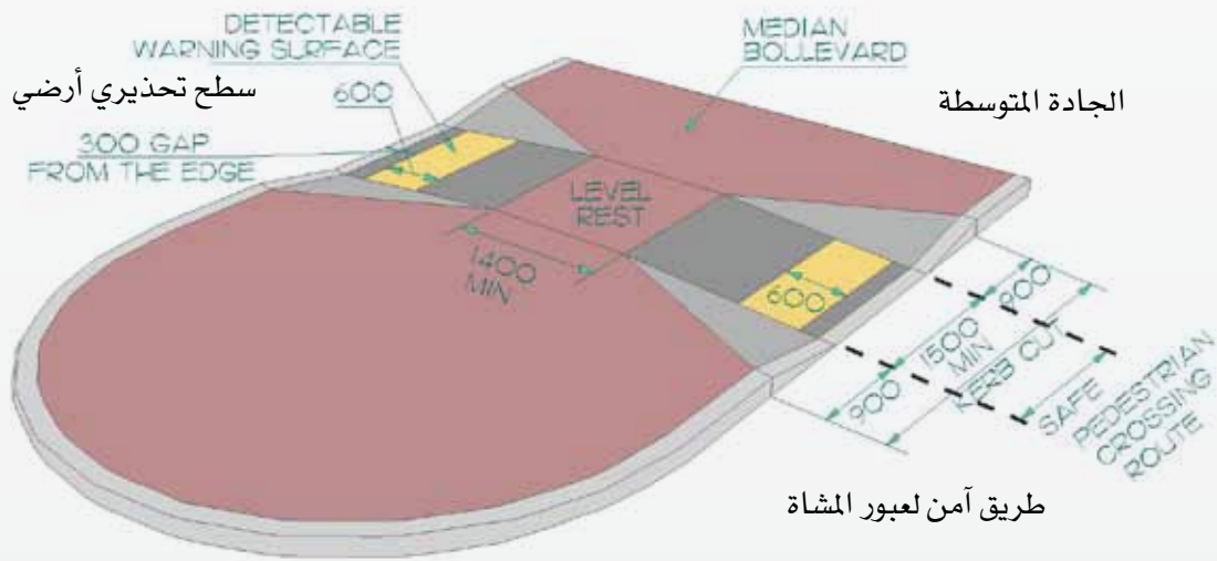
شكل ٦٨: جزيرة تقسيم عريضة مرتفعة
