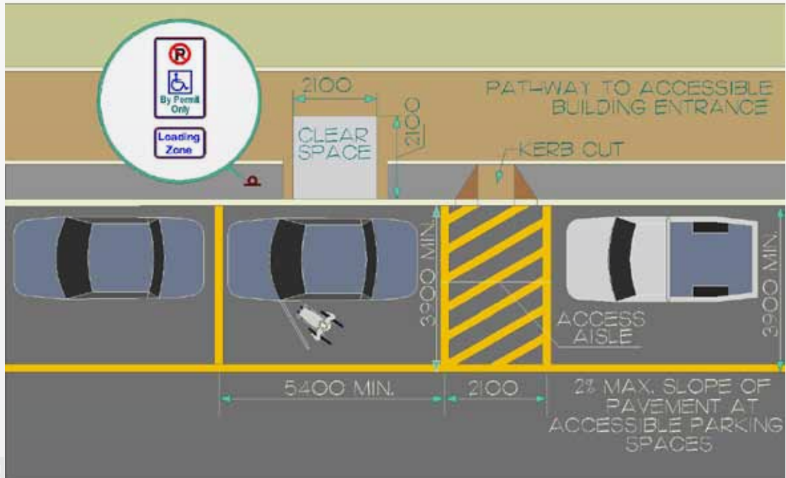
شكل ٧٢: المواقع العمودية
