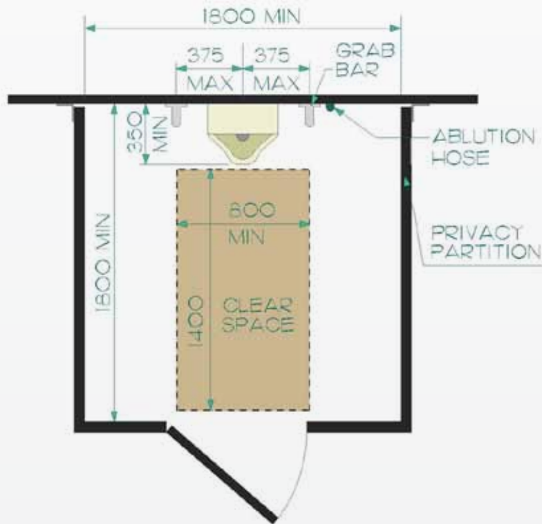
شكل ١٥١: حجرة المبال
