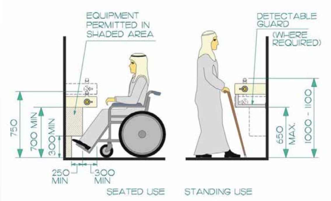
شكل ٢٠٠: أبعاد النافورة
