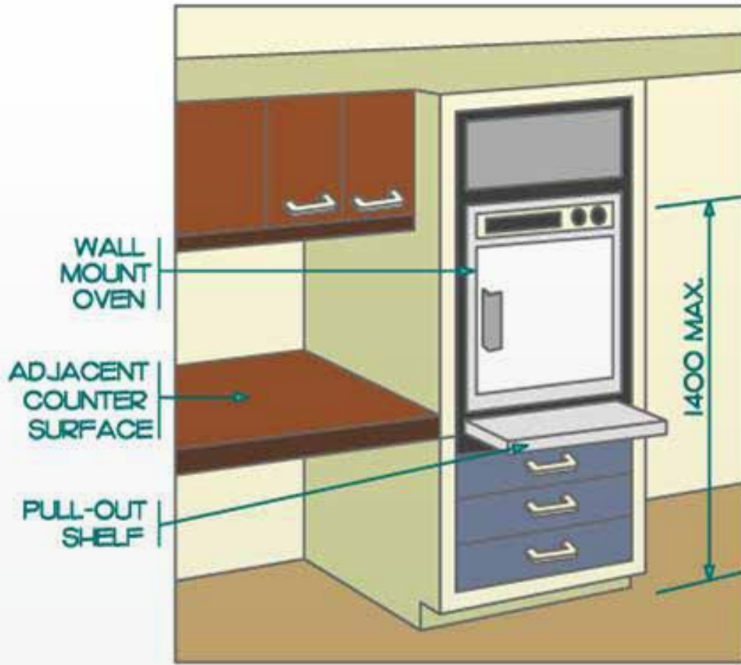
شكل ١٦٨: موقد داخل الحائط
