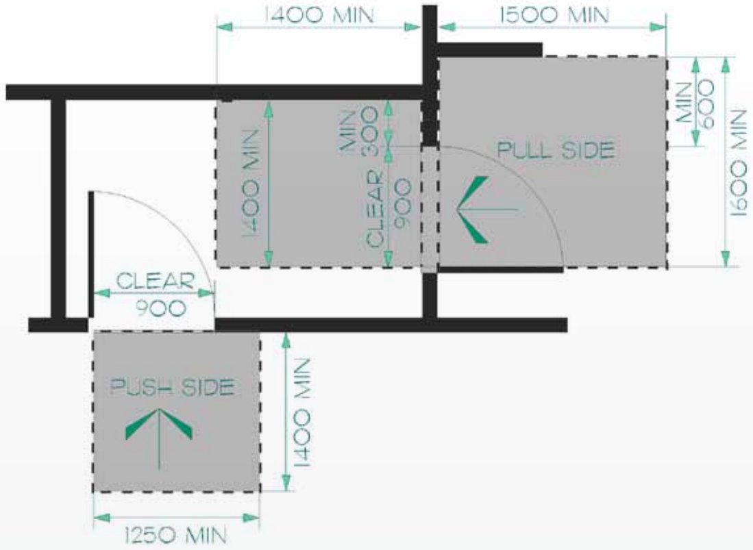
شكل ١٢١: مساحة الدوران عند الأبواب في سلسلة
