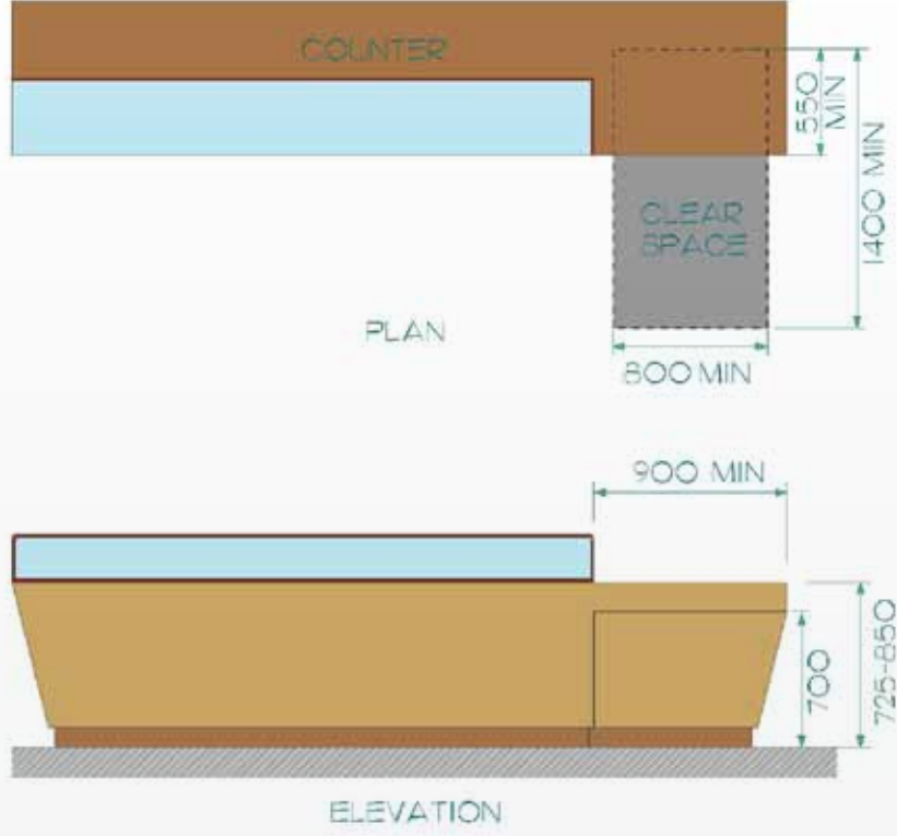
شكل ١٨٤: مكتب الخدمة
