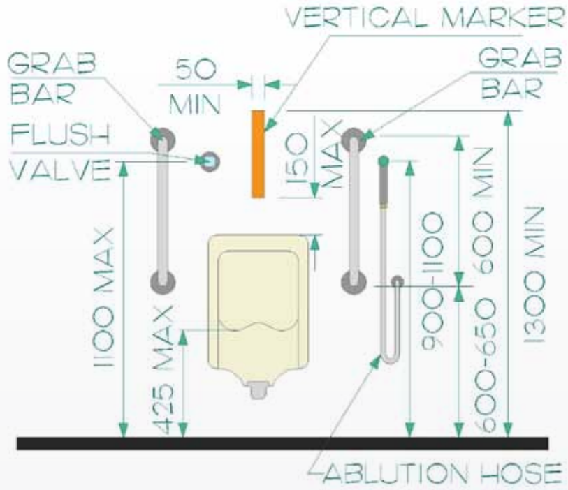
شكل ١٥٢: ارتفاع المبوالة
