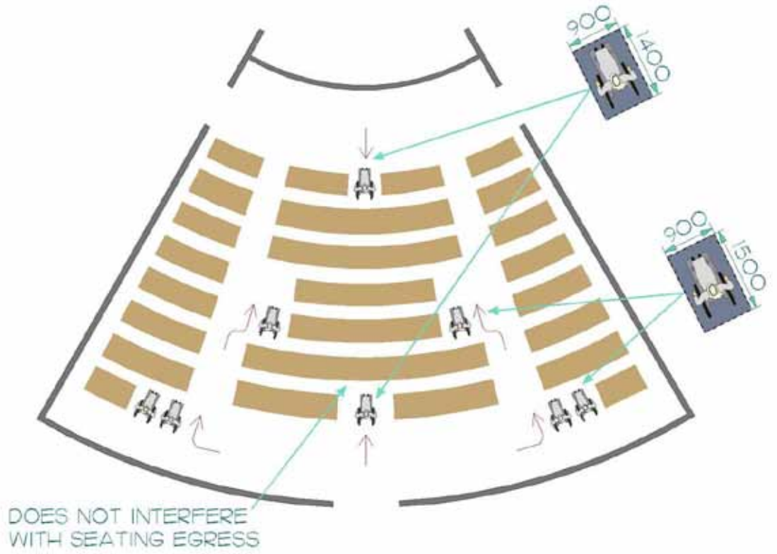
شكل ١٨٩: توزيع أماكن المشاهدة سهلة الوصول
