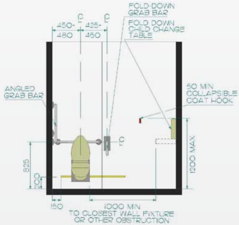
شكل ١٤٠: غرفة حمام ملائمة لاستخدام الجنسين
