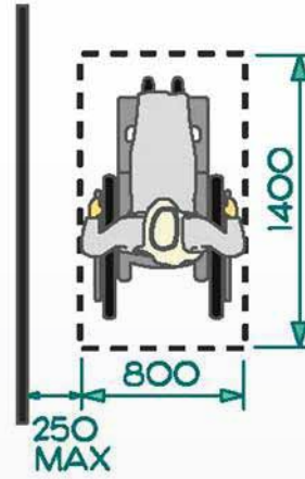
شكل رقم ١٩: فراغ الوصول الجانبي، المسافة القصوى للكرسي المتحرك
