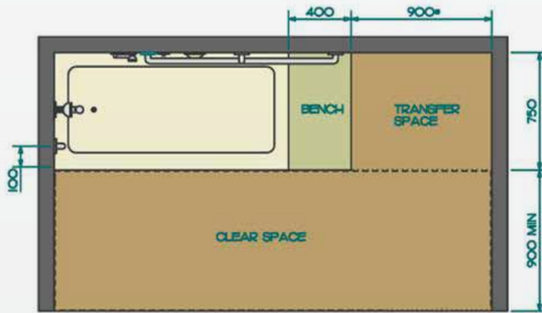
شكل ١٥٥: حوض الاستحمام
