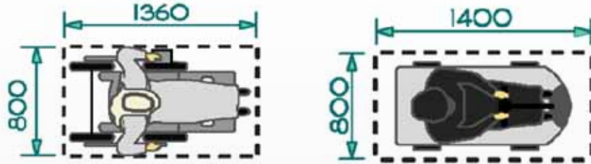
شكل رقم ٩: الفراغ لشخص يستخدم كرسيًا متحركًا كهربائيًا شكل رقم ١٠: الفراغ لشخص يستخدم سكوتر التنقل
