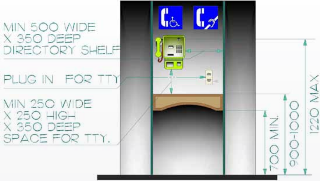
شكل ٢١٤: الهواتف
