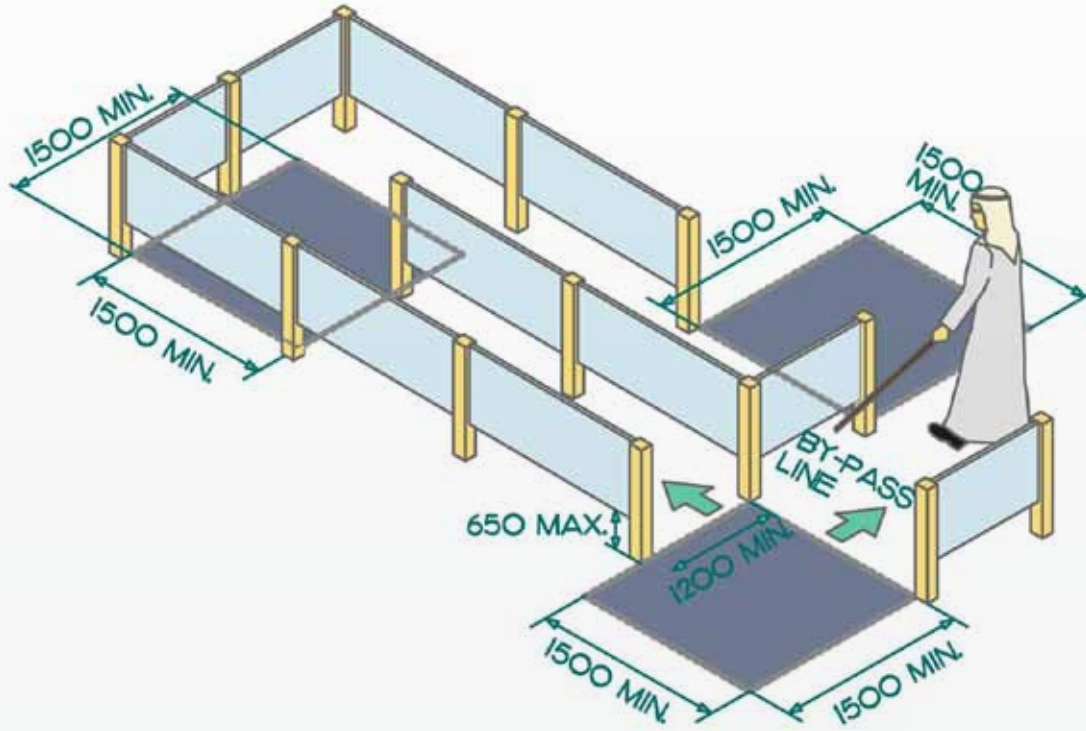
شكل ١٨٥: منطقة الانتظار
